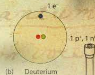
(b) Deuterium
